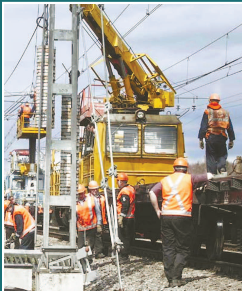
Монтаж опытных участков контактной сети для скорости движения 250 км/ч на участке Калашниково - Лихославль Октябрьской железной дороги
